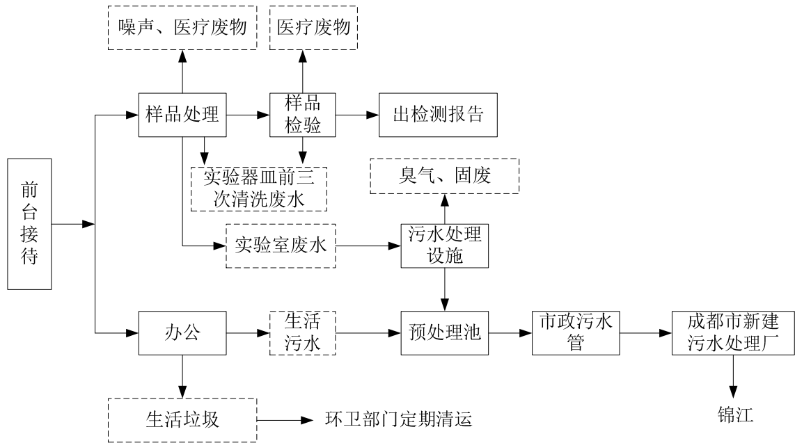
图 2-1 营运期流程及产污位置图
